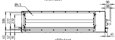
előlnézet
