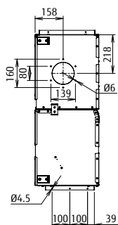
oldalnézet (B)
