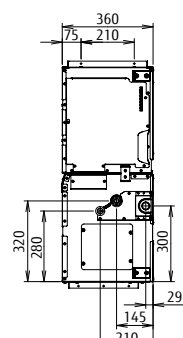
oldalnézet (J)
